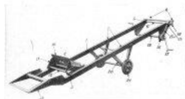
Fig. 18. — Bomba mobile
